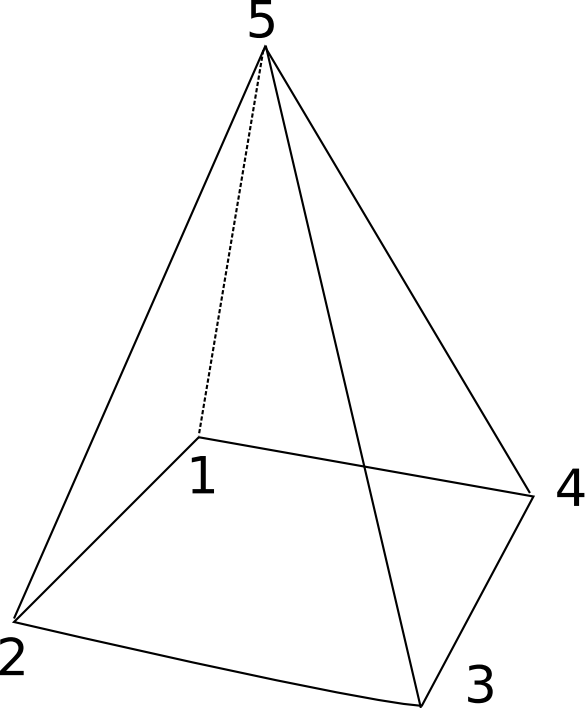
Pyramid
